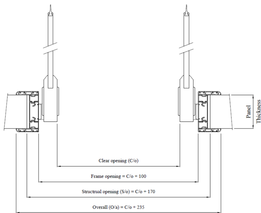
Double Leaf Door
